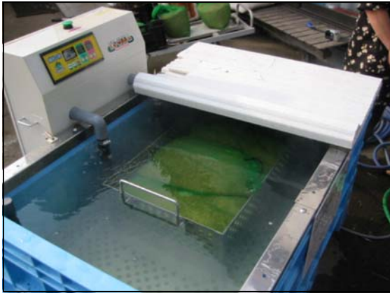
種籾の温湯消毒 約60℃×10分
